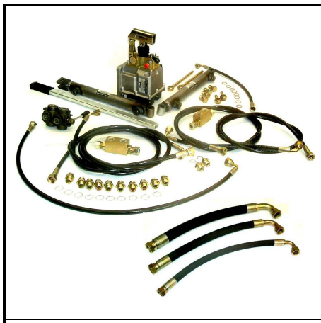
Kit Tubi flessibili raccordati Hose fittings
